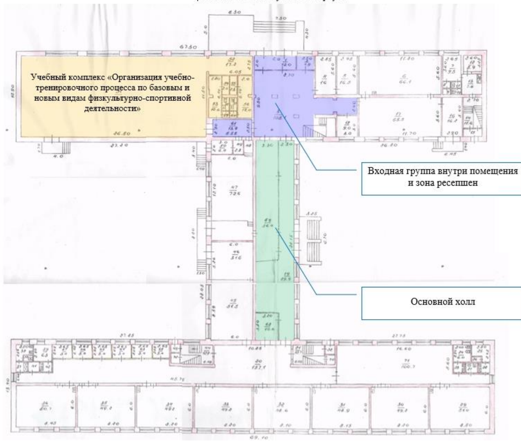
План-схема 1 этажа учебного корпуса
