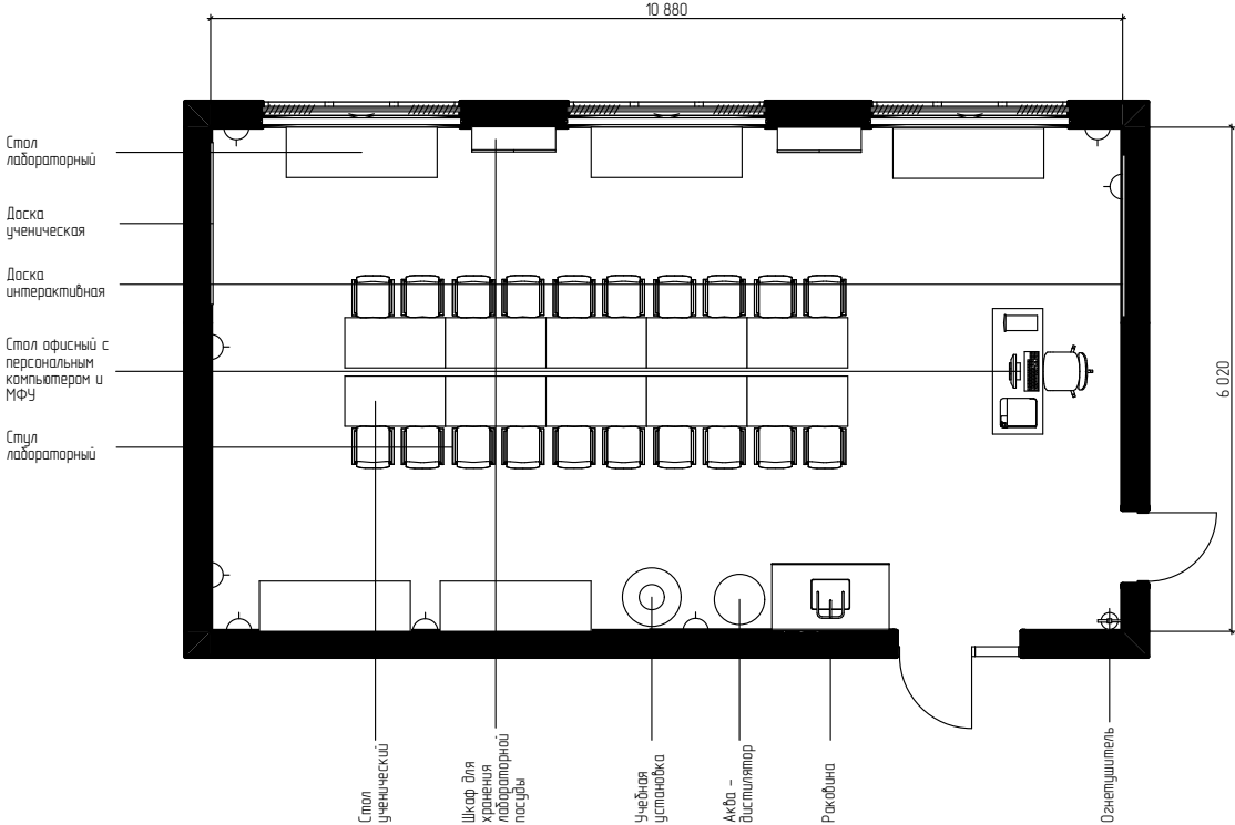
План расстановки и маркировки мебели и оборудования М 1:100 Зона 11. Зона под вид работ Производство напитков. Литер А1
