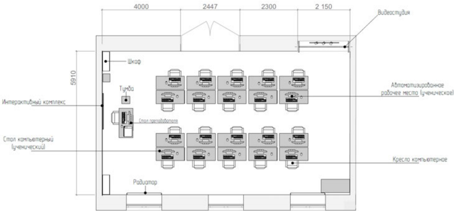
План расстановки и маркировки мебели и оборудования М 1:00 Зона 8. Интерактивное обучение 2 эт. лит. А1
