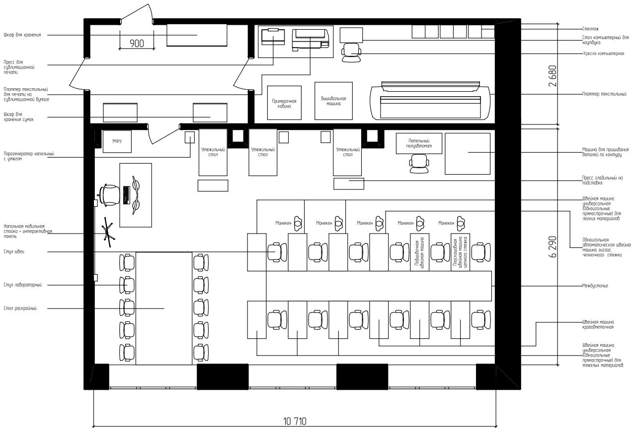
План расстановки и маркировки мебели и оборудования М 1:100 Зона 3. Зона под вид работ Текстильный дизайн 2 эт. лит. Е
