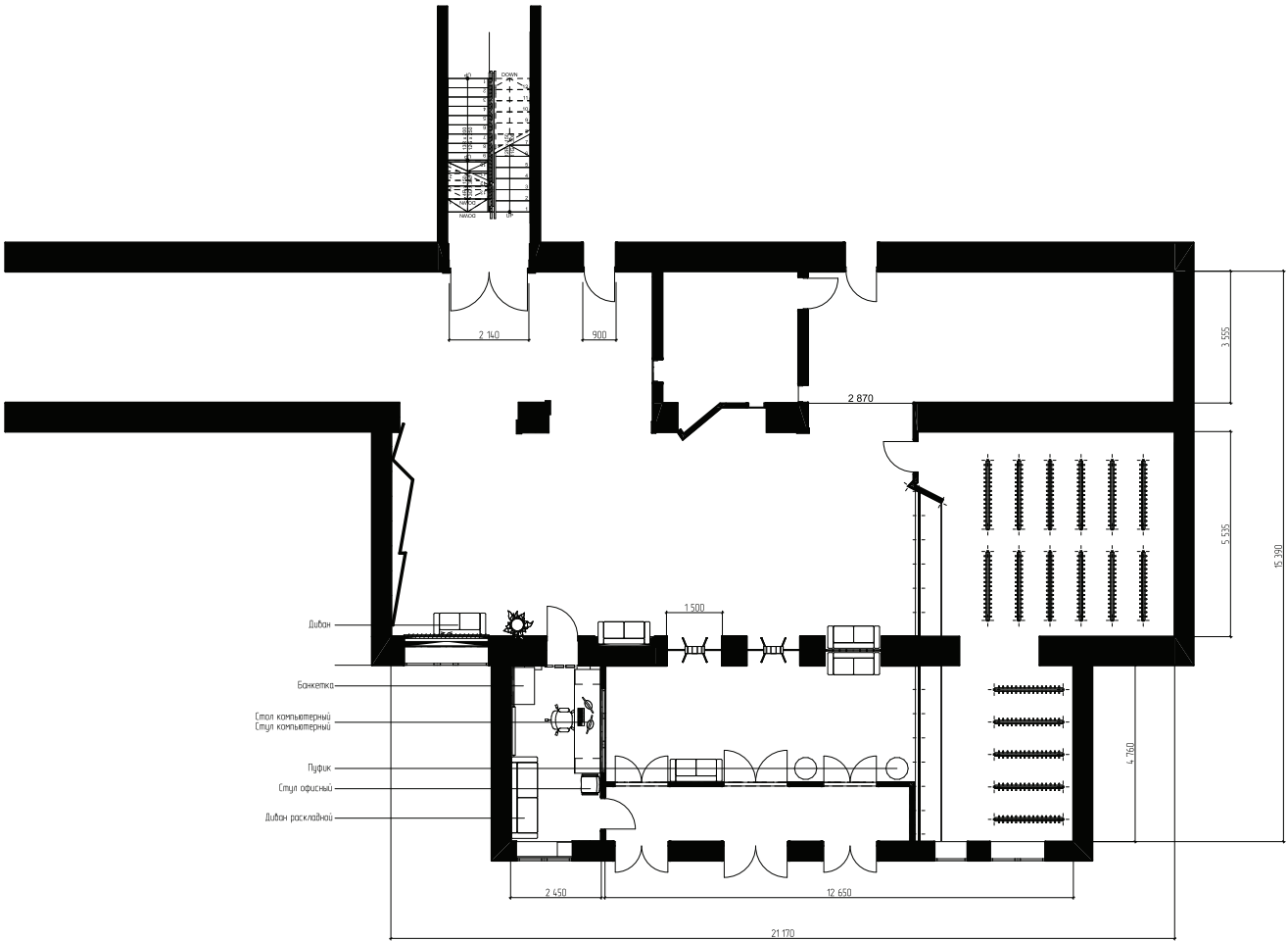
План фойе 1 этажа М:200
