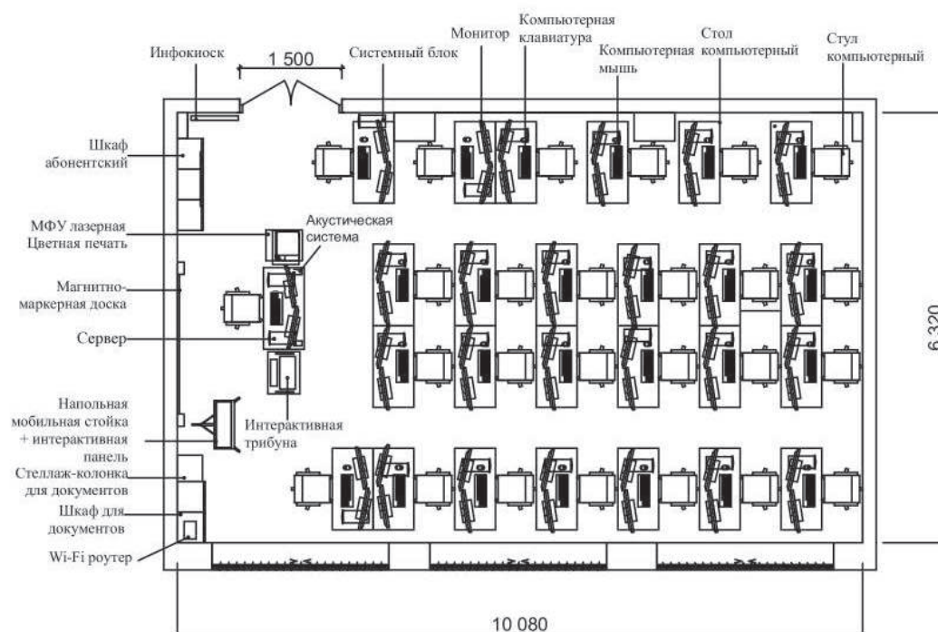
План расстановки и маркировки мебели и оборудования М 1:100 Зона 1. Веб-дизайн 2 эт. лит. Е
