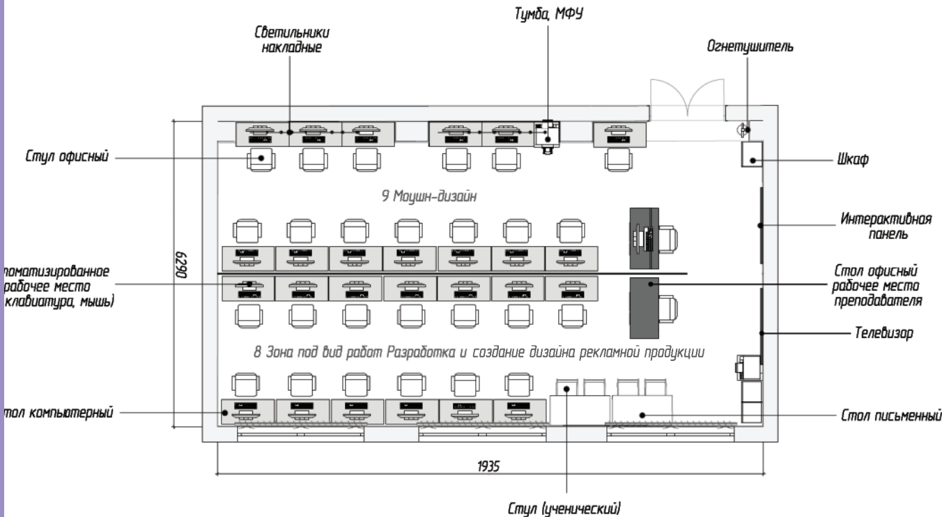
План расстановки и маркировки мебели и оборудования М:100 8 Зона под вид работ Разработка и создание дизайна рекламной продукции 9 Моушн-дизайн 2 эт. лит. Е
